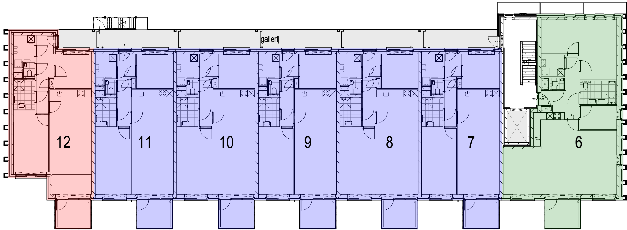
Eerste verdieping
